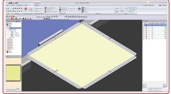
MBend'e aktarıldıktan sonra sac montaj parçası
